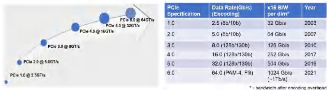
图表121： PCIe 不同代际的性能参数表
