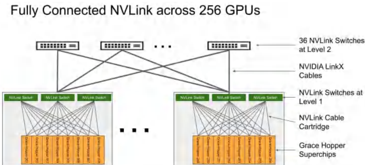
图表123： GH200 的网络连接示意图
