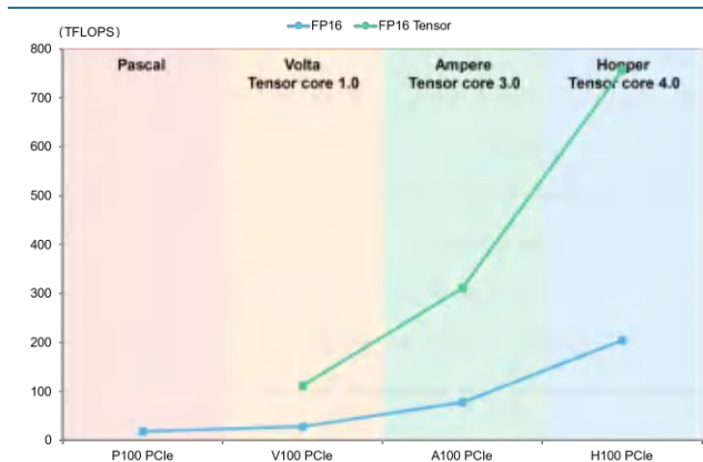
图表22： FP16 Tensor 算力快速增长
