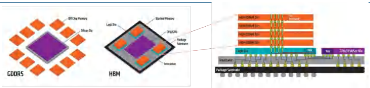
图表26： GDDR 与 HBM 差异
