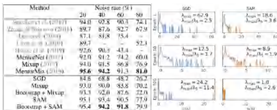
图表171： SAM 提升了模型对标签噪声的稳健性，并优化了模型训练效率
