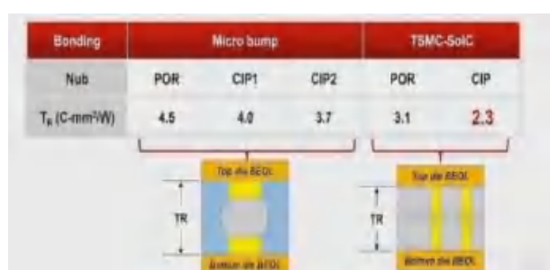
图表91: SoIC 具有更优异的热性能表现
