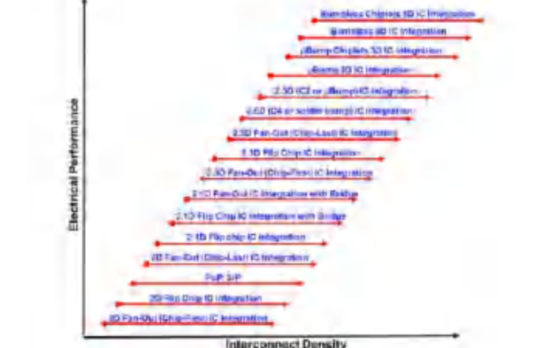
图表71： 先进封装依据互连密度和性能排名
