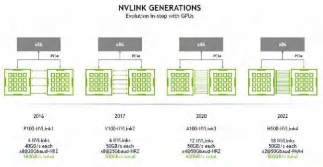
图表120： NVLink 不同代际的升级 Roadmap
