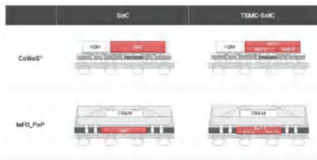
图表89：SoIC 与 InFO_PoP、CoWoS 联合应用
