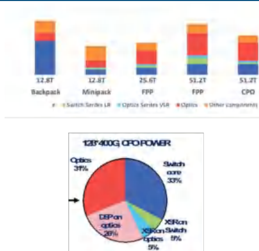
图表140： CPO 所降低的功耗拆分示意图
