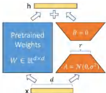
图表177: LoRA 只调试低秩的 A、B, 预训练权重保持不变
