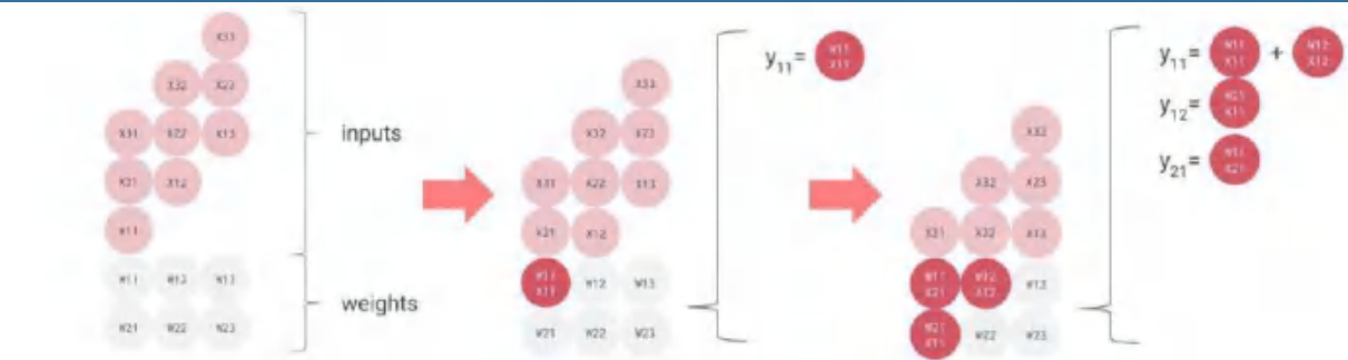
图表35： 脉动阵列运行矩阵乘法的示意图
