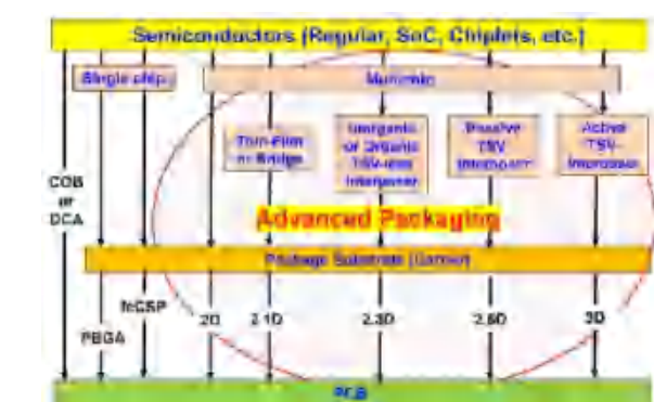
图表70： 先进封装的层次
