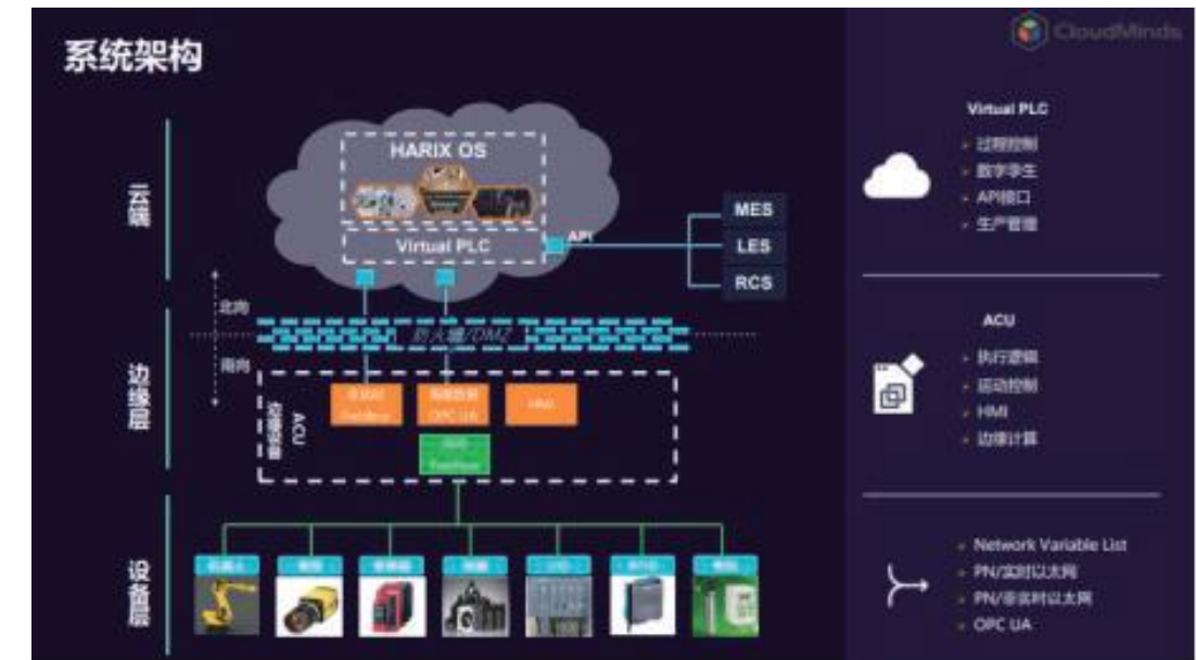
达闼云化PLC系统架构
